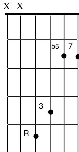
G Maj7b5
