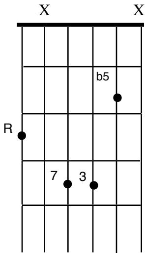
G Maj7b5
