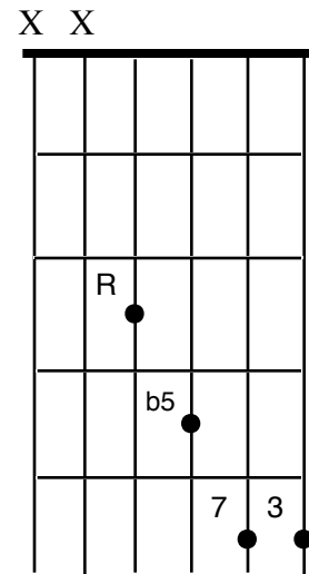
FMaj7b5
